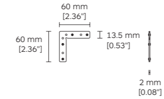
2G54 L-bracket (For 2ST3, 2ST5, 2ST8 & 2STA)
