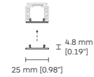
2G54 L-bracket (For 2ST3, 2ST5, 2ST8 & 2STA)
